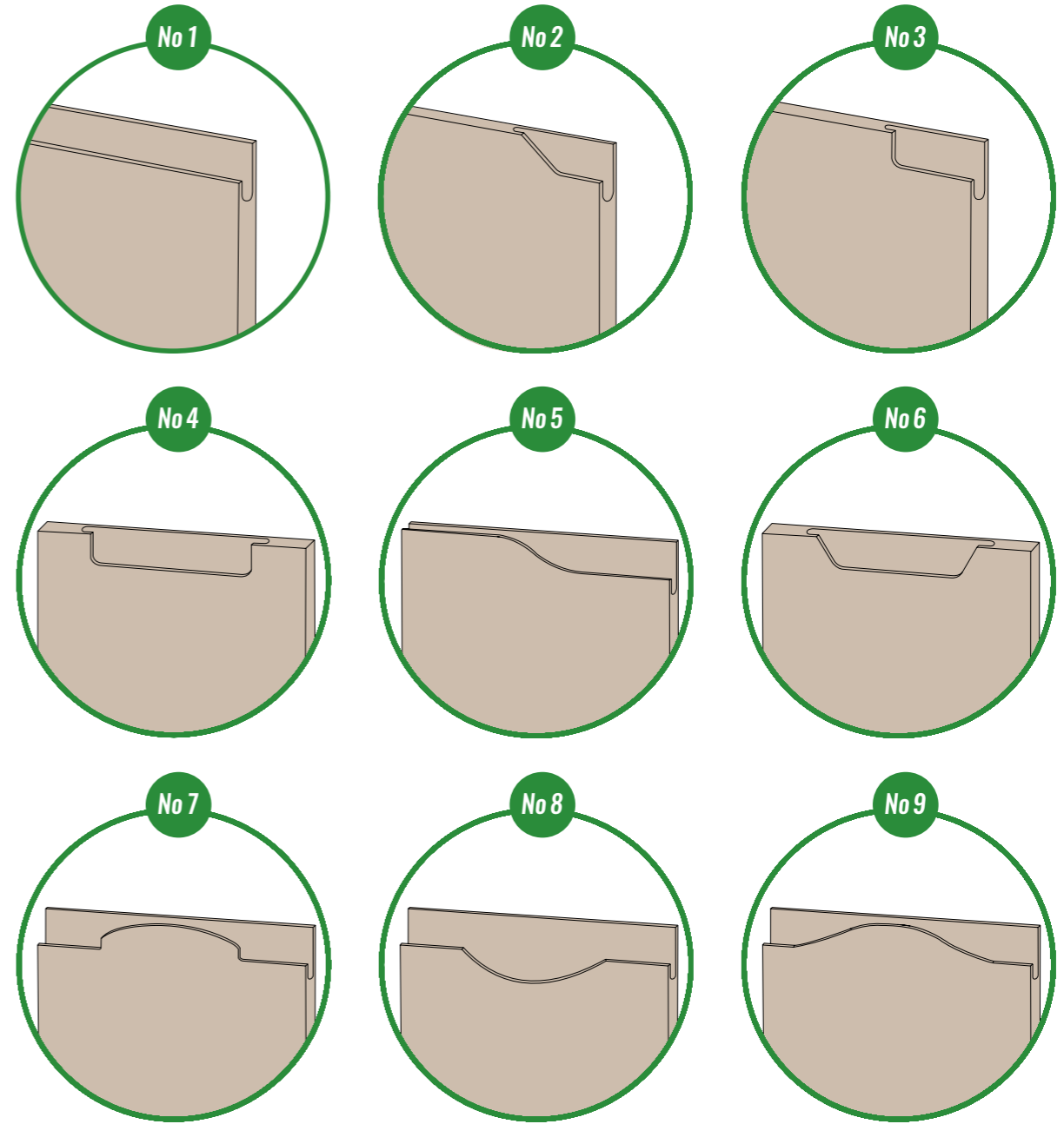
Профиль (сечение), толщина и возможное исполнение
