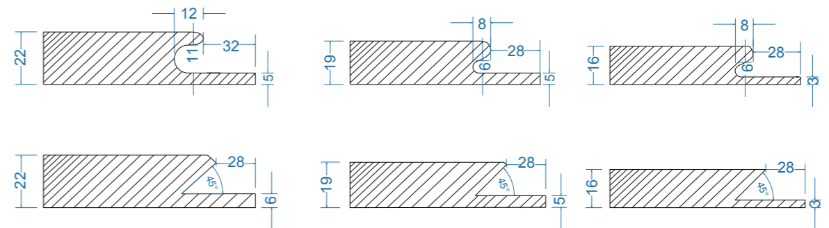
Профиль (сечение), толщина и возможное исполнение
